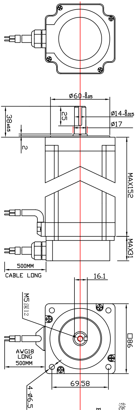
机械尺寸 Dimension
